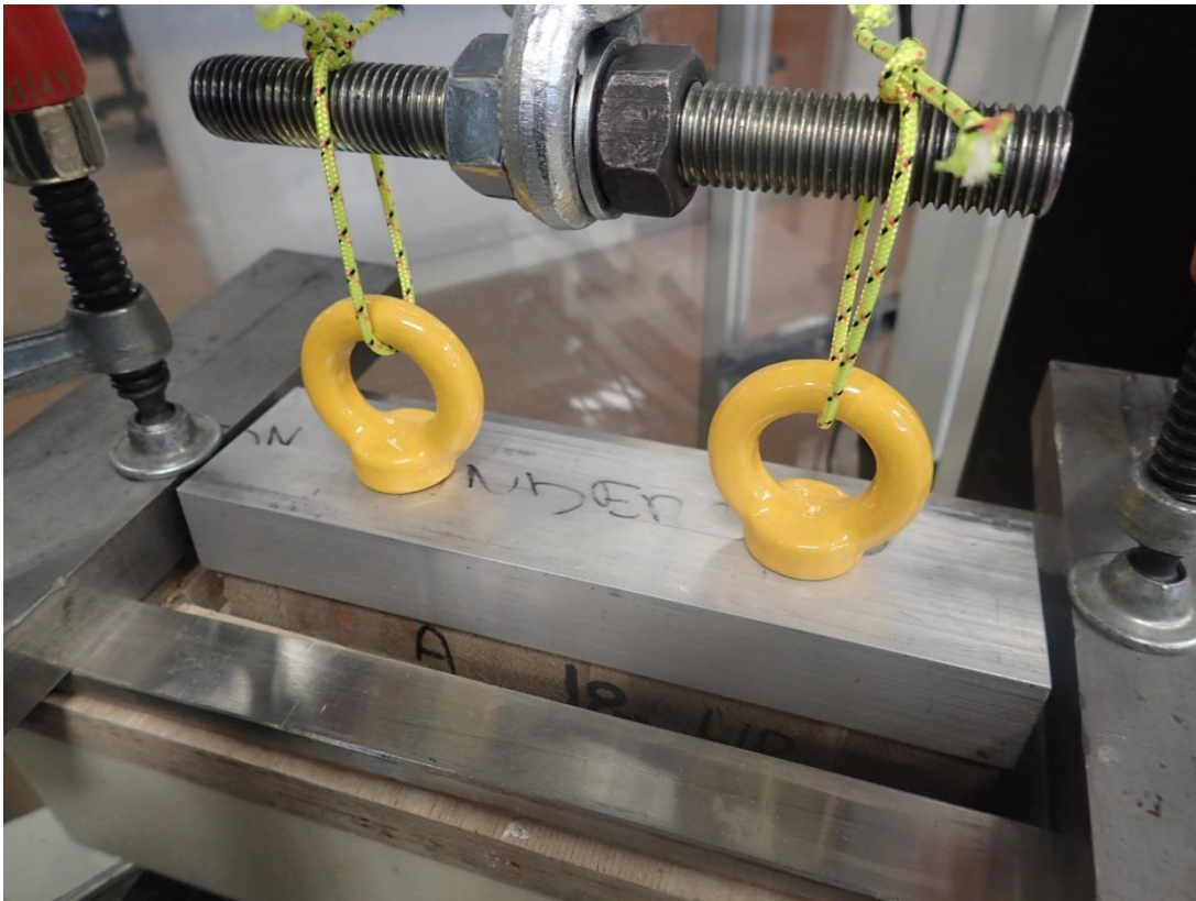
Foto 3. Aftrækstest med aluminiumsklodser.
